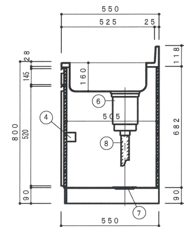
側面断面図 1/15
