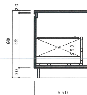
側面断面図 1/15
