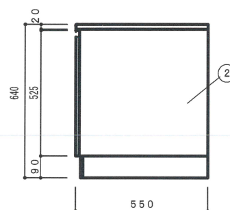
側面立面図 1/15
