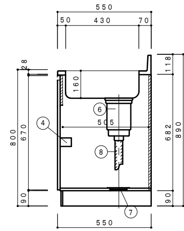
側面断面図 1/15
