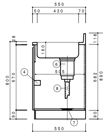
側面断面図 1/15
