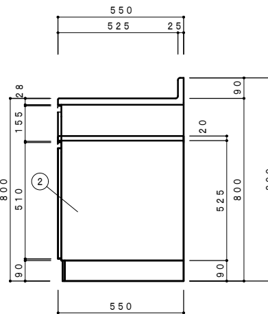
側面立面図 1/15
