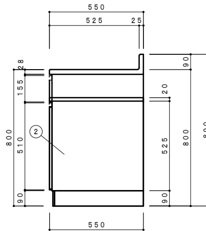
側面立面図 1/15
