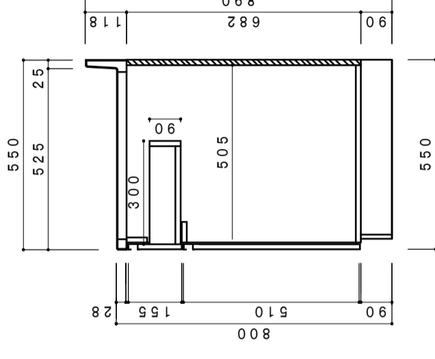
側面断面図 1/15
