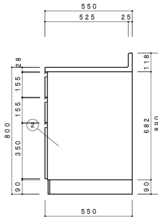
側面立面図 1/15
