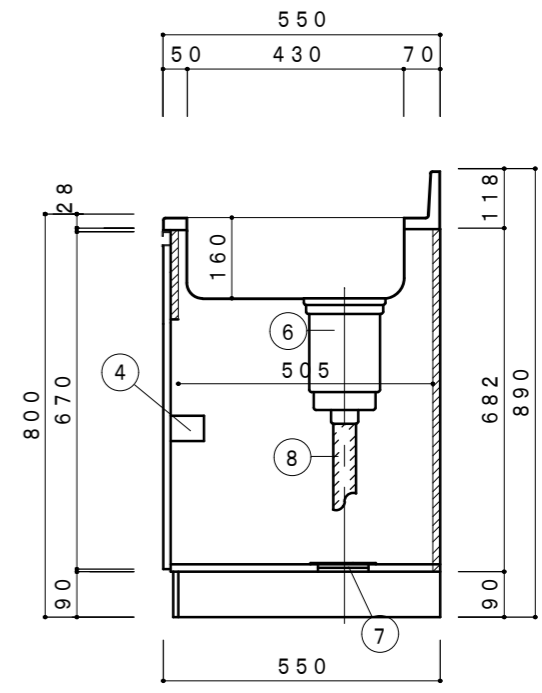
側面断面図 1/15
