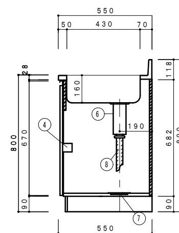
側面断面図 1/15
