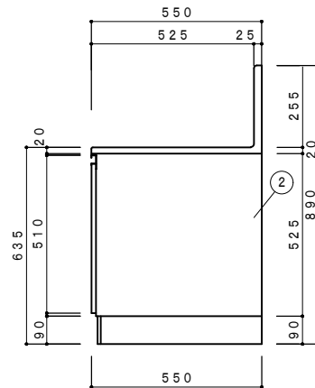
側面立面図 1/15
