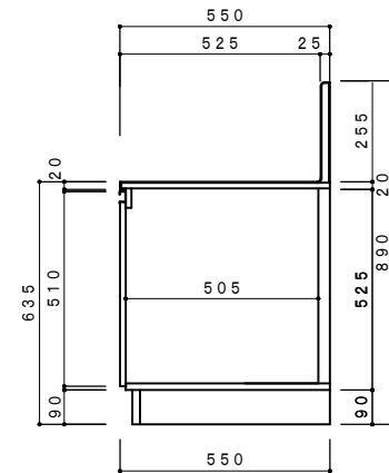
側面断面図 1/15
