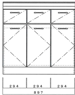
正面図 1/20
