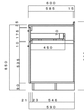
側面断面図 1/20
