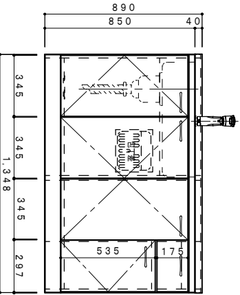
正面図 1/20
