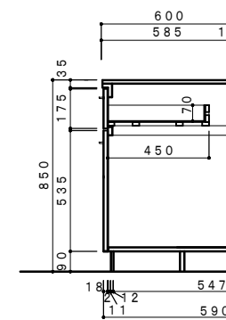
側面断面図 1/20
