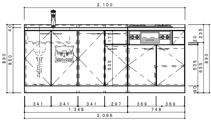
正面図 1/20
