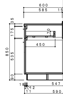
側面断面図 1/20
