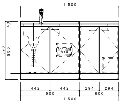
正面図 1/20
