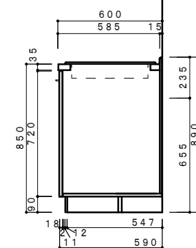
側面断面図 1/20
