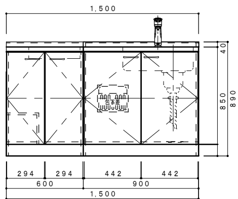
正面図 1/20
