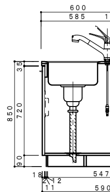
側面断面図 1/20
