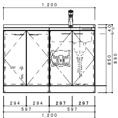
正面図 1/20
