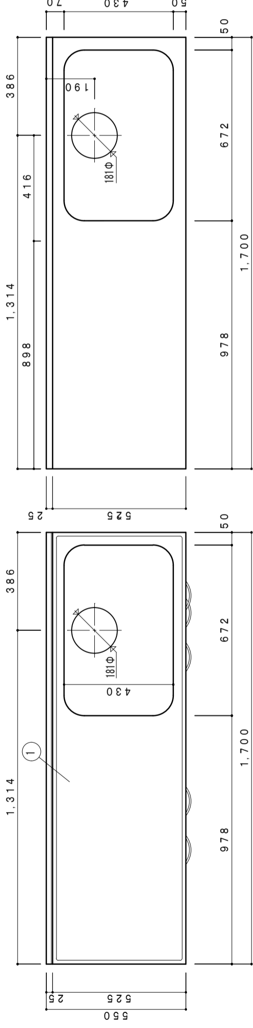
天板開口寸法 1/15
