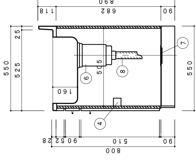
側面断面図 1/15
