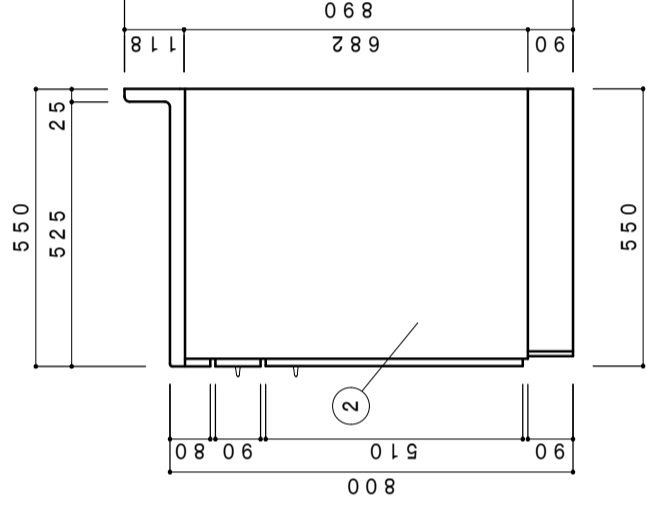
側面立面図 1/15
