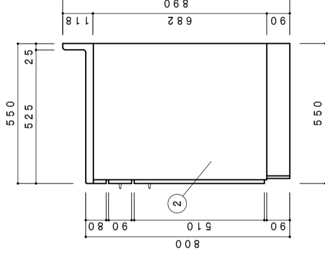
側面立面図 1/15
