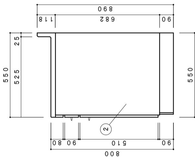
【側面立面図 1/15】
